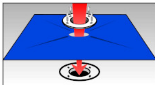
Positionnement de la pièce destinée à l'imperméabilisation élastique des syphons (300 m x 300 m)
